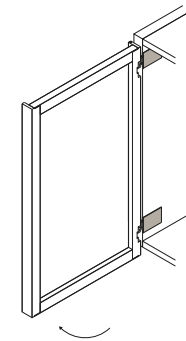
DETTAGLIO CERNIERA / HINGE DETAIL
